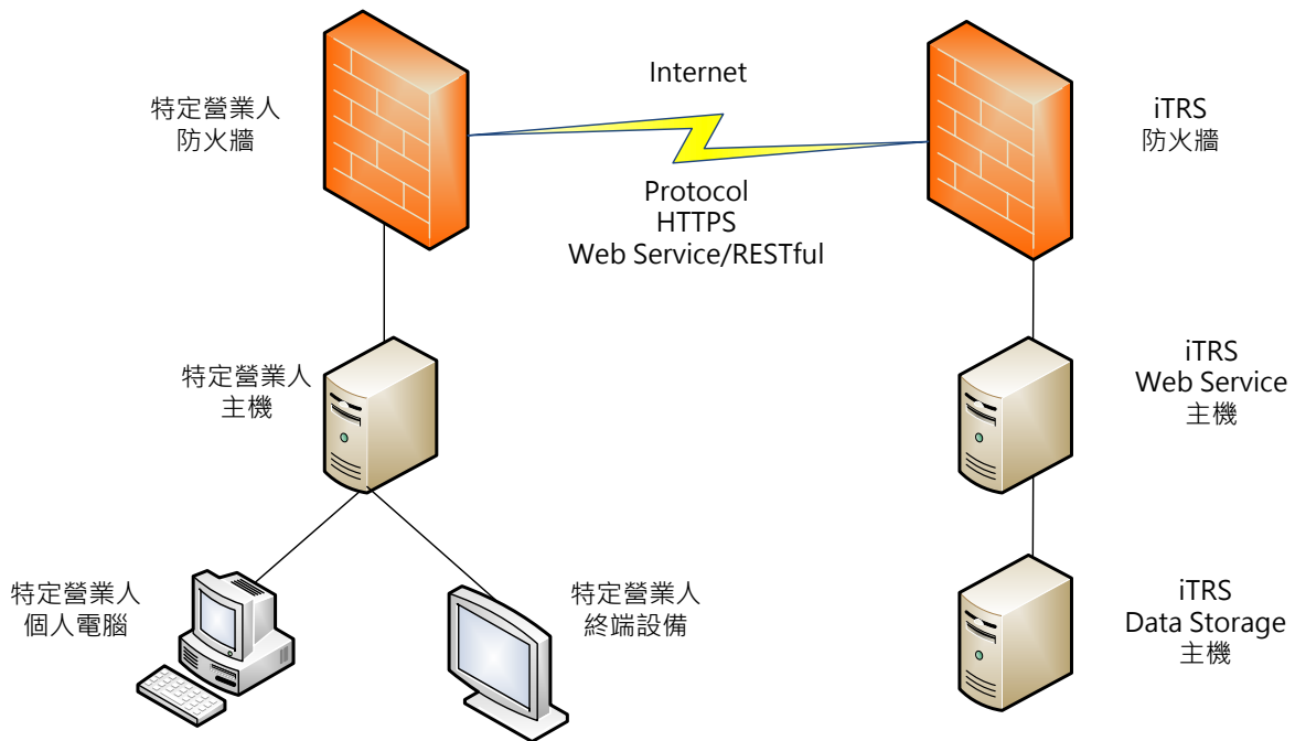
【圖1】系統架構圖
